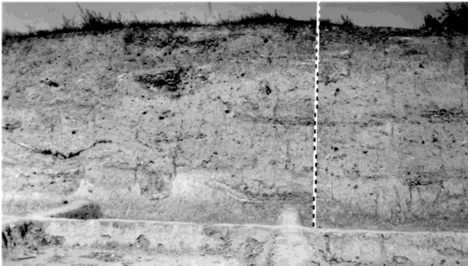
Обр. 1. Тел Казанлък. Тахиметричен план с квадратна мрежа и зона на рондела (1). Стратиграфски профил (2).
