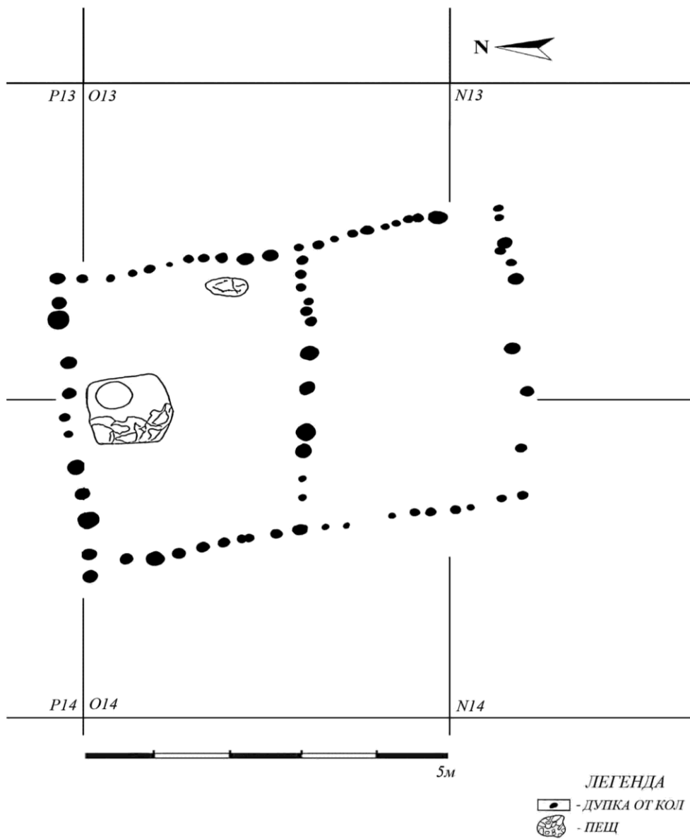
Обр. 9. Тел Казанлък. IX строителен хоризонт. План на жилище 3. Среден неолит. Период Протокараново III.
