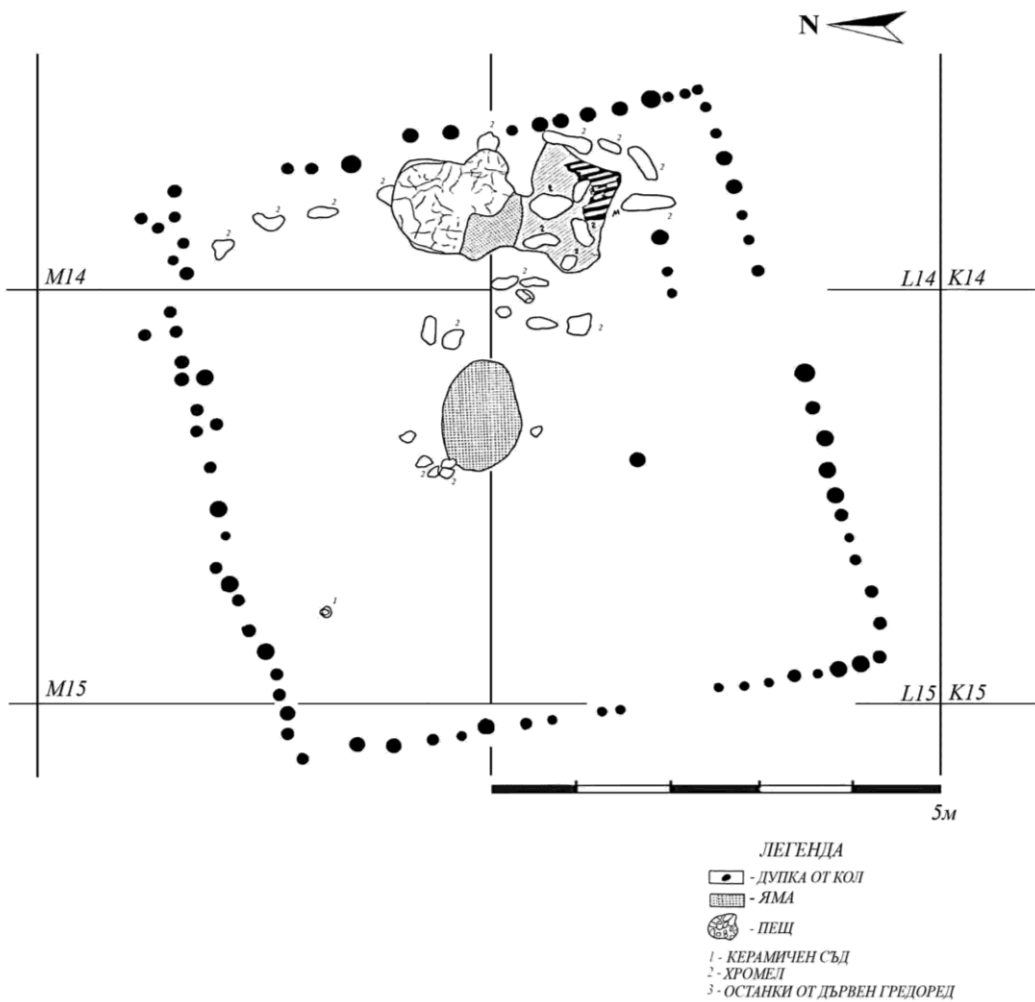
Обр. 7. Тел Казанлък. IX строителен хоризонт. План на жилище 1. Среден неолит. Период Протокараново III.
