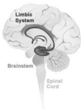
Обр. 6 Лимбалният дял в мозъка на човека и художественото му стилизиране като лимб
