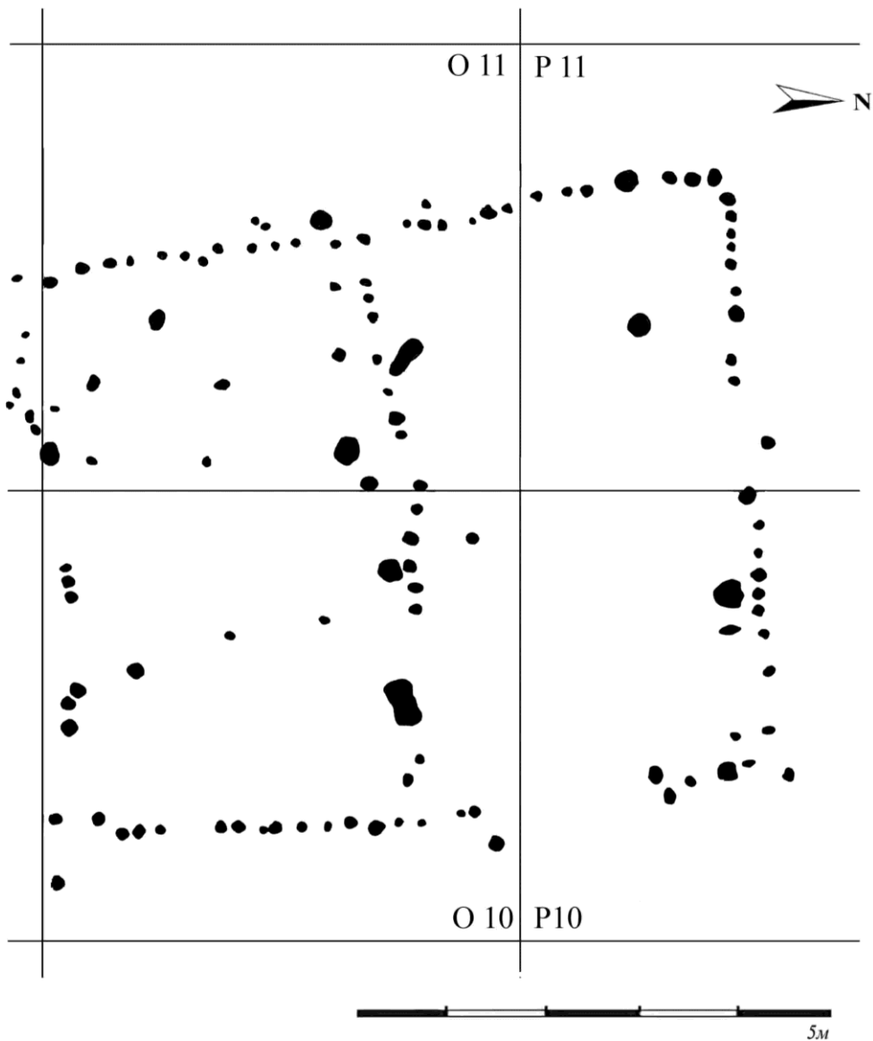
Обр. 12. Тел Казанлък. III строителен хоризонт. План на жилище 3. Късен неолит. Период Караново III.
