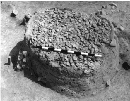
Обр. 2. Тел Казанлък. X строителен хоризонт. Гроб на дете (1). Подове на жилища (2). Основи на пещи (3).
