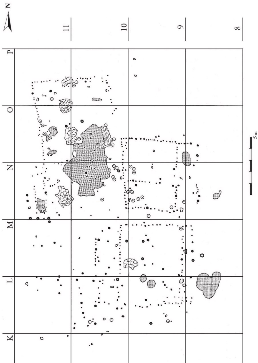
Обр. 10. Тел Казанлък. III строителен хоризонт. Структури и съоръжения, документирани в източната половина на неолитното селище.
